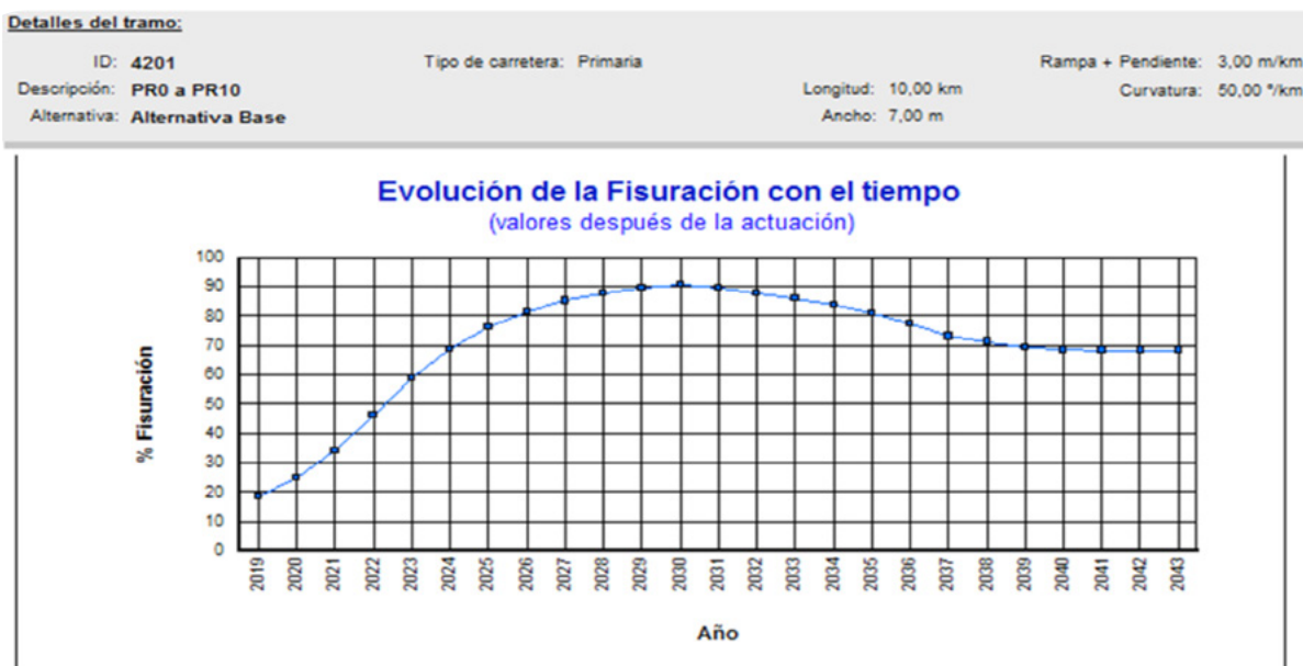
▲ Imagen 8.25 | Simulación de deterioro de pavimento flexible con alternativa base en HDM4.
