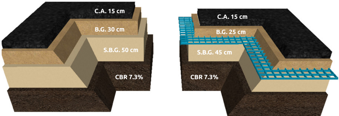
▲ Figura 6.11 | Optimización de espesores mediante Geomalla a) estructura inicial b) estructura con Geomalla.
