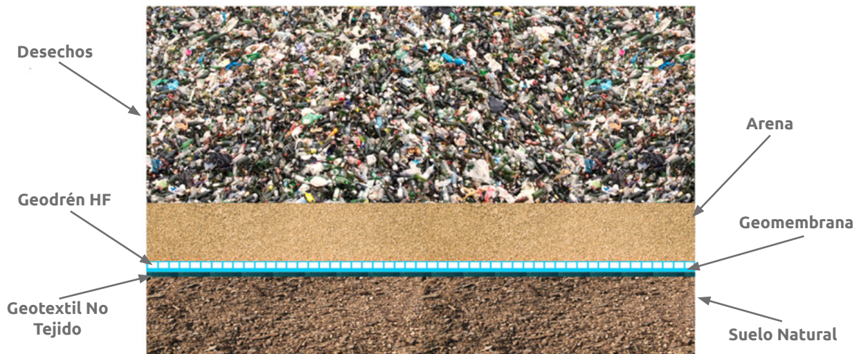
▲ Figura 10.12 | Aplicación del Geodrén HF en rellenos sanitarios.
