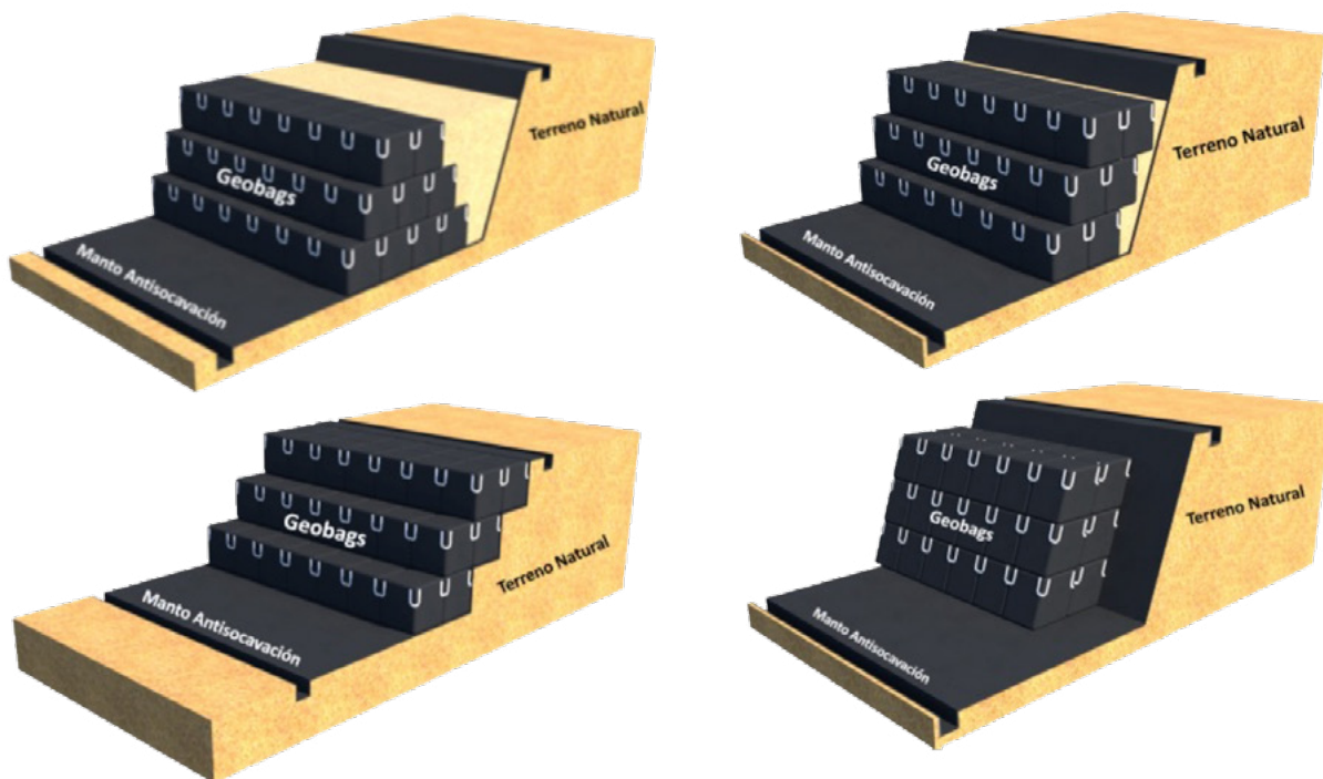
▲ Figura 17.1 | Configuraciones geométricas estructuras de protección con Geobags.
