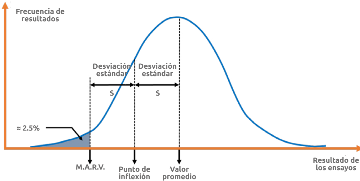
▲ Figura 2.7 | Relaciones relativas de diferentes valores usados en la especificación de los Geosintéticos.
