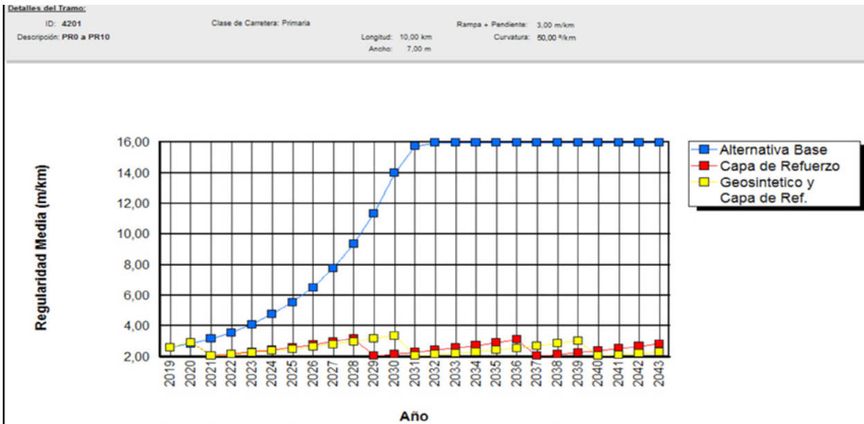
▲ Imagen 8.28 | Simulación de IRI de las 3 alternativas de conservación en HDM4.
