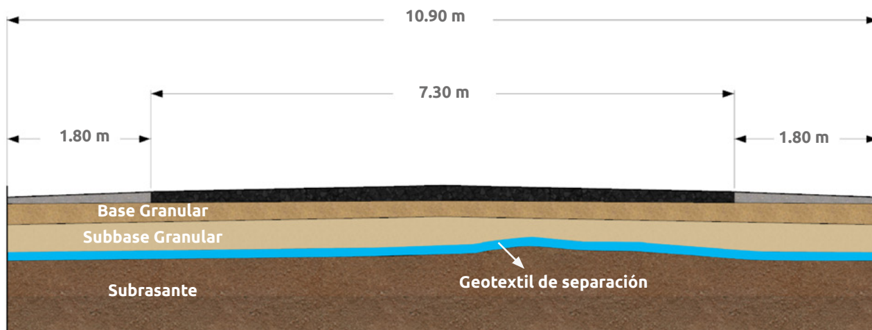
▲ Figura 5.4 | Sección transversal del ejemplo.
