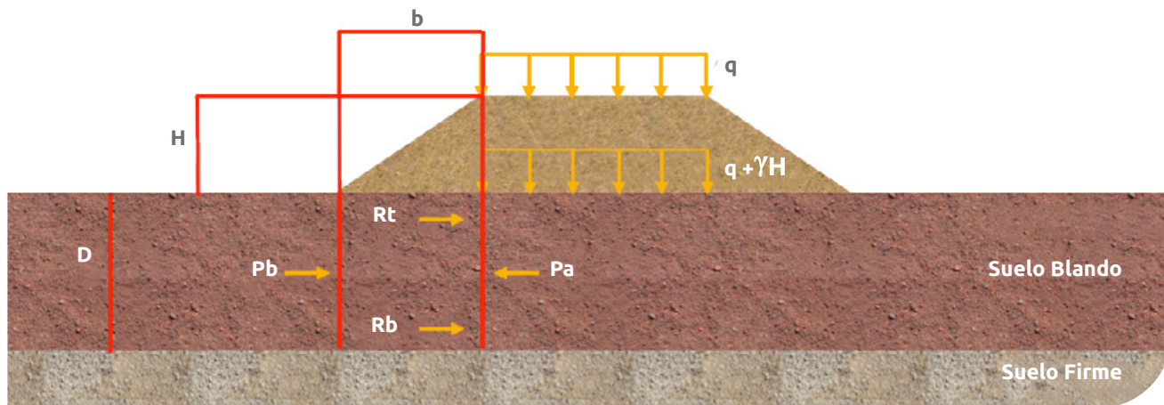
▲ Figura 13.10 | Expulsión del suelo blando.
