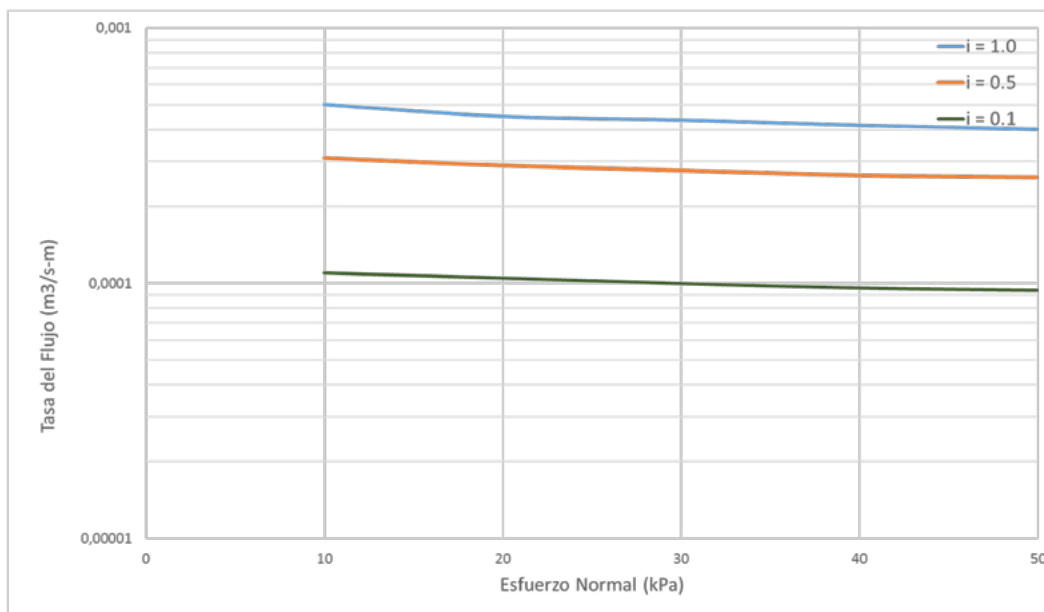
▲ Figura 10.17 | Tasa de flujo en función del esfuerzo normal y el gradiente hidráulico Geodrén Planar i=1.0 , i=0.5 y i=0.1 – Sentido Transversal.
