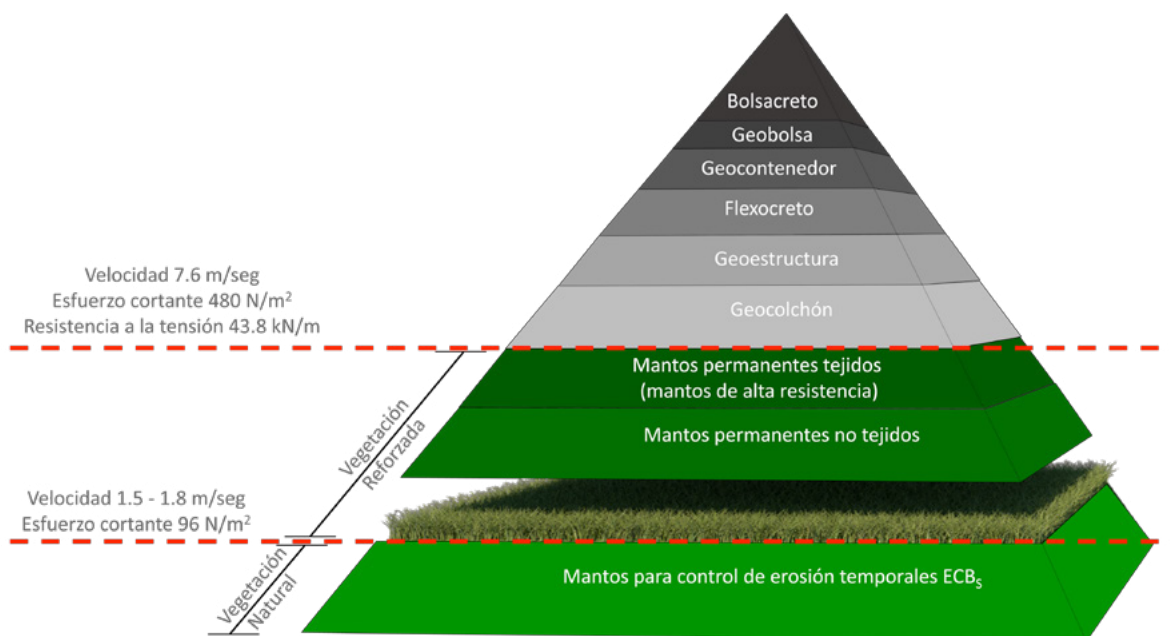
▲ Figura 16.1 | Pirámide de erosión y soluciones con Geosintéticos.
