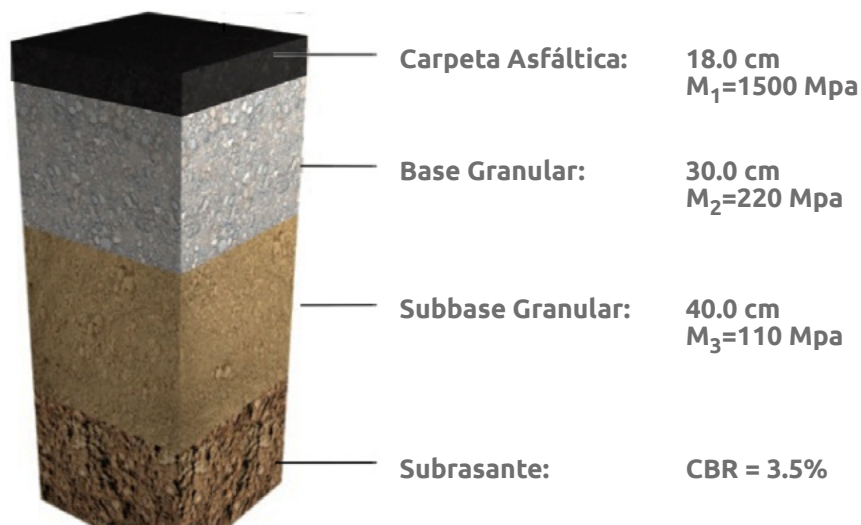
▲ Figura 7.14 | Estructura del ejemplo.
