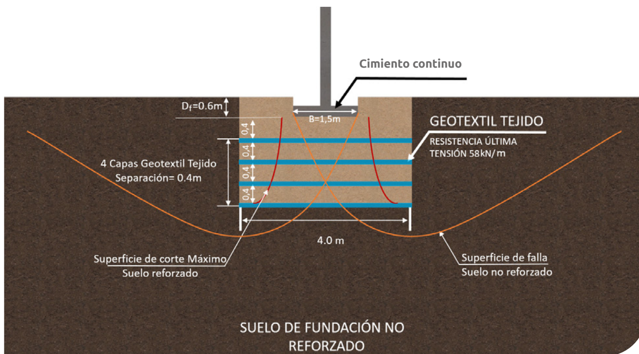
▲ Figura 14.13 | Esquema de refuerzo de la fundación.
