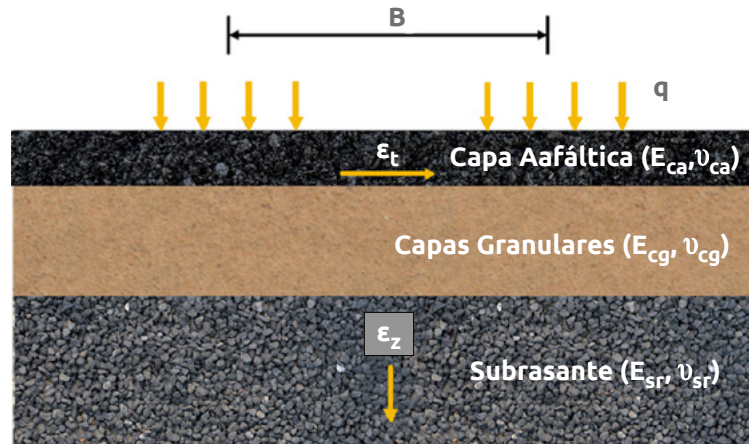
▲ Figura 7.10 | Modelo de análisis racional de pavimentos.
