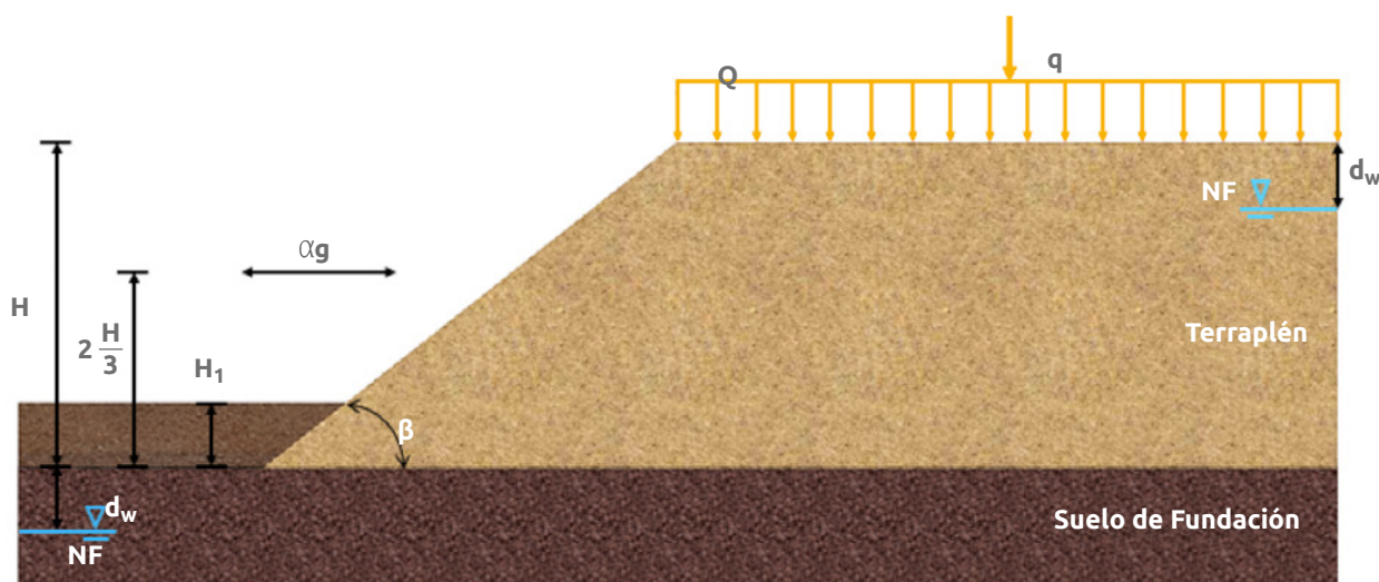
▲ Figura 13.1 | Esquema terraplén.
