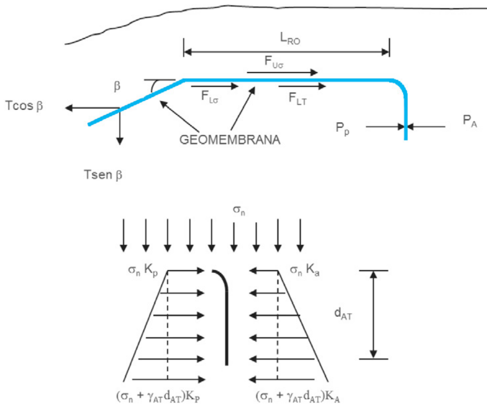
▲ Figura 15.3 | Sección transversal de la longitud de desarrollo de una Geomembrana con zanja de anclaje y fuerzas actuantes.
