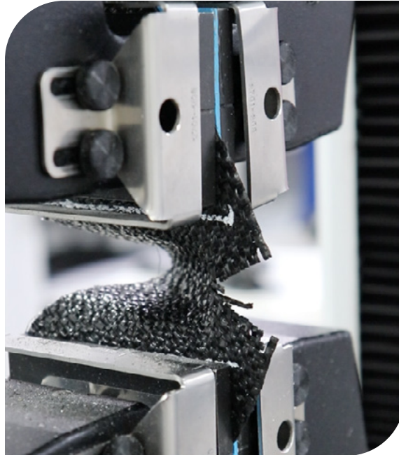
▲ Fotografía 2.23 | Inicio ensayo rasgado trapezoidal.
