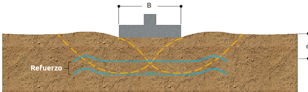
▲ Figura 14.4 | Falla por pullout.
