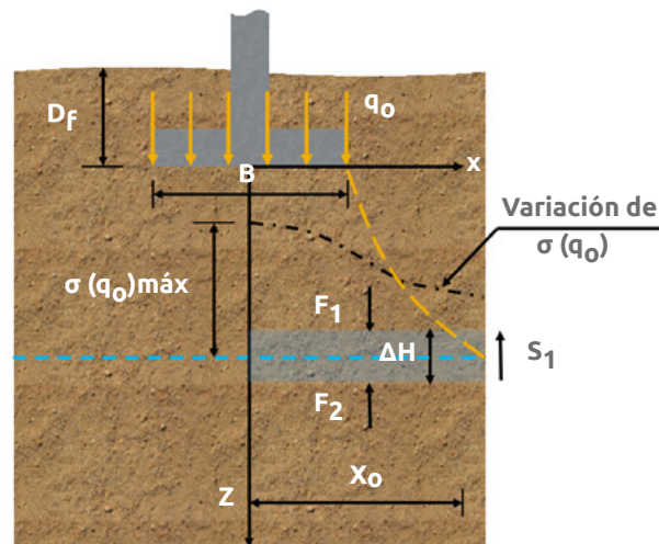
▲ Figura 14.8 | Fuerzas actuantes en cimentaciones no reforzadas.
