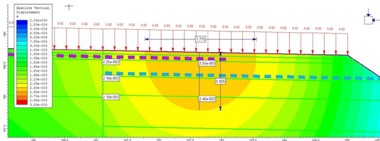
▲ Imagen 8.20 | Desplazamientos verticales en ampliación de calzada con refuerzo de Geomallas en la junta. Sección transversal. Línea punteada superior: Geomalla de Fibra de Vidrio. Línea punteada inferior: Geomalla Biaxial Coextruida para granulares.
