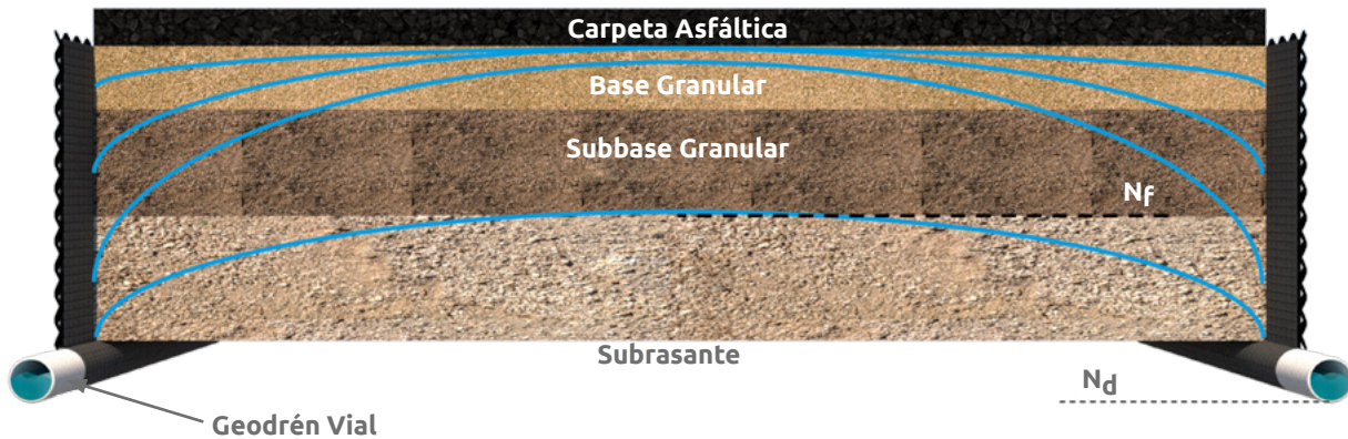
▲ Figura 10.19 | Geodrén Vial (con tubería perforada).
