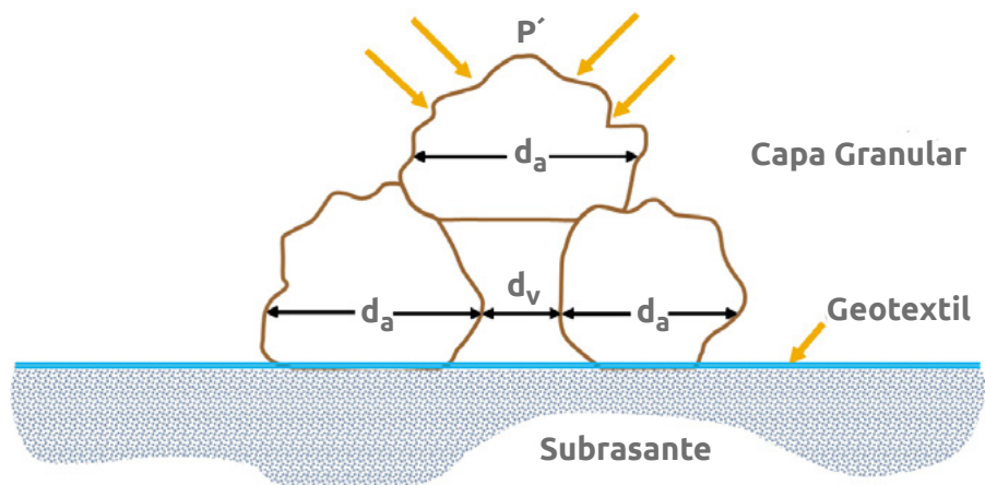
▲ Figura 5.2 | Geotextil de separación- Resistencia a la tensión (GRAB).
