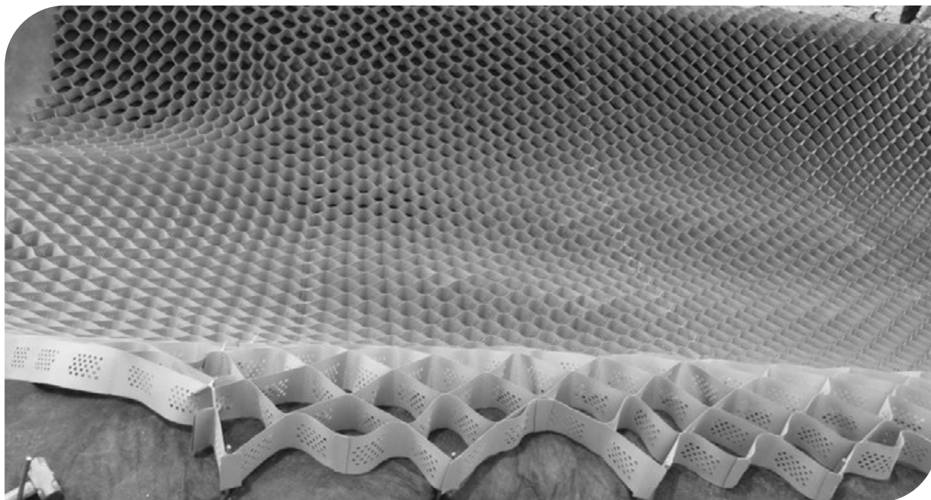
▲ Fotografía 17.48 | Extensión del panel de la Geocelda.
