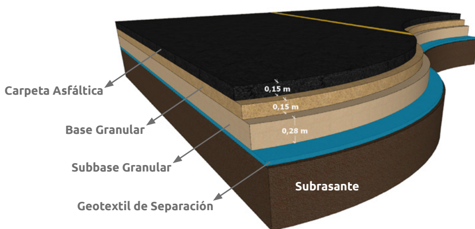
▲ Figura 5.8 | Estructura con Geotextil de separación.
