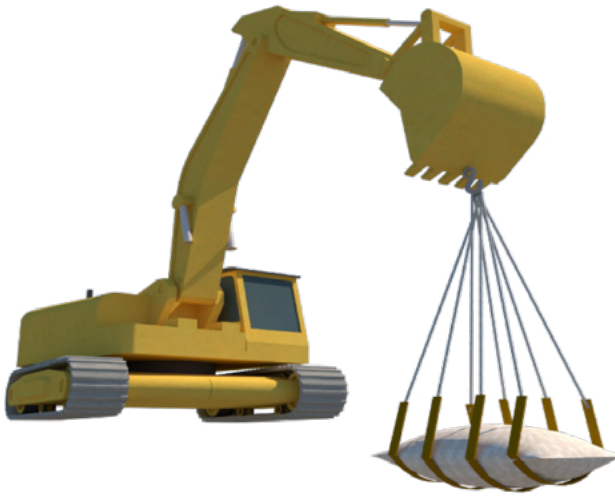
▲ Figura 17.23 | Izado con eslingas.
