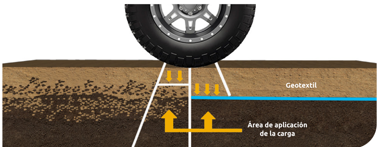
▲ Figura 4.1 | Separación de capas granulares y suelo de sitio.
