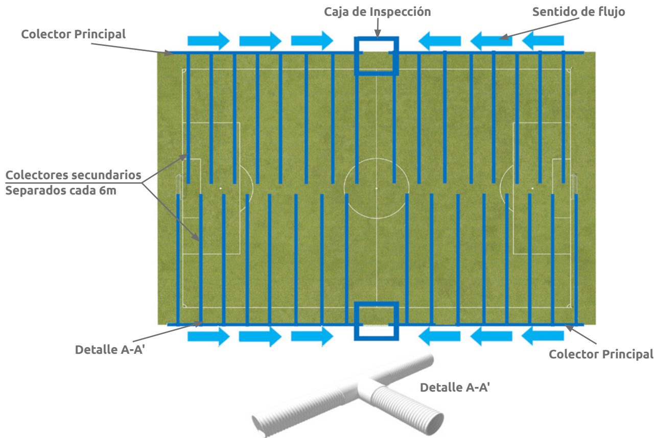
▲ Figura 10.22 | Distribución esquemática de los colectores principales y los colectores secundarios.
