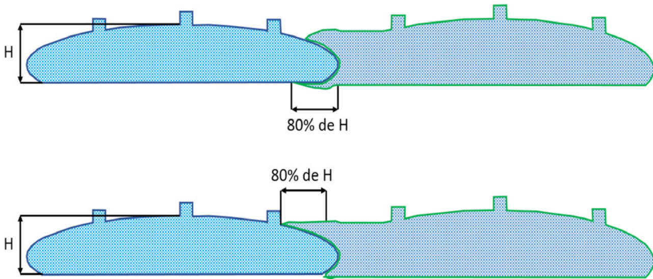
▲ Figura 17.9 | Tipos de traslapos para Geotextile Tubes.
