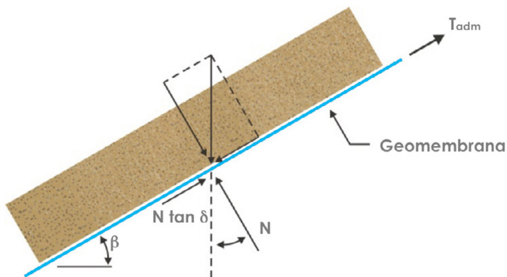
▲ Figura 15.2 | Fuerzas actuantes con suelos de cobertura sobre la Geomembrana de recubrimiento, con profundidad de suelo constante.
