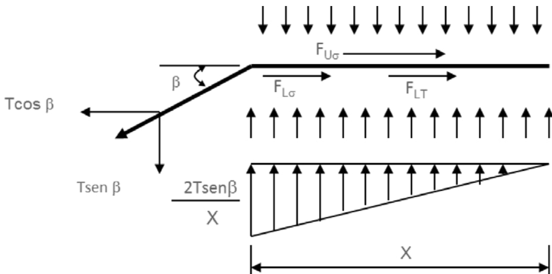
▲ Figura 15.1 | Modelo de diseño utilizado para calcular el espesor de la Geomembrana.
