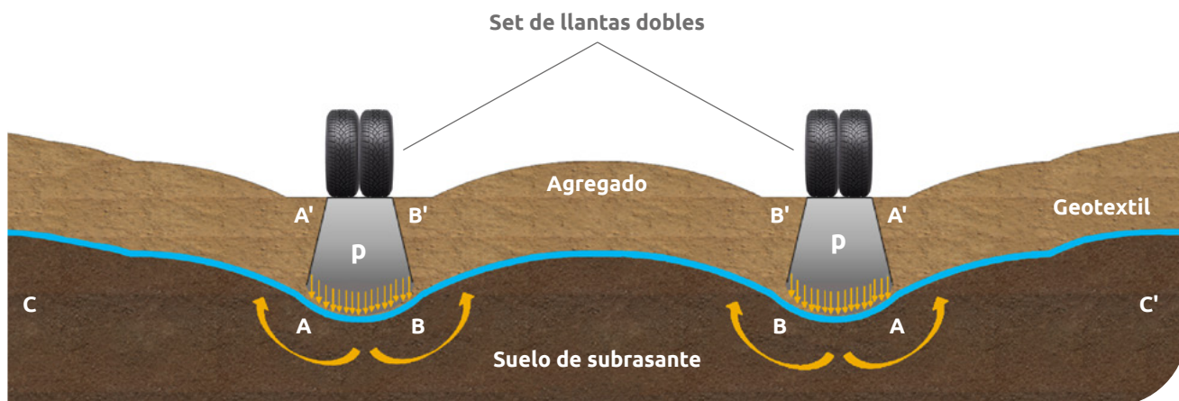
▲ Figura 4.2 | Efecto membrana.
