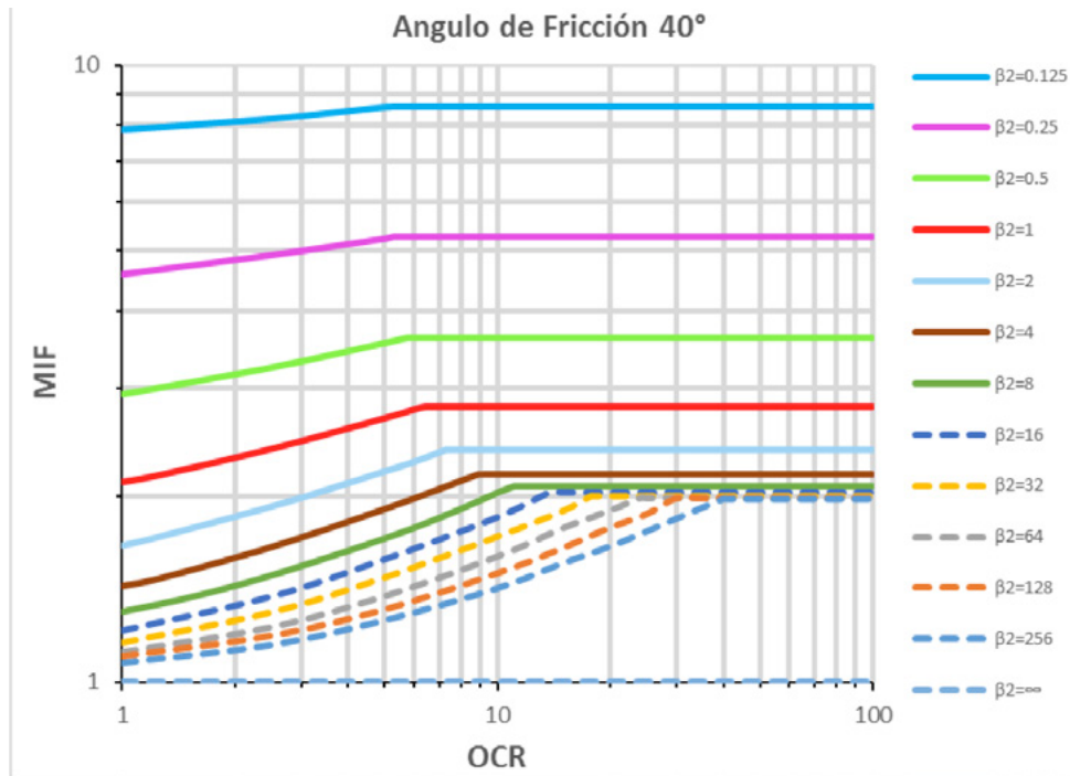
▲ Figura 7.8 c | Gráficos para la determinación de MIF en capas de suelo reforzadas con Geoceldas.
