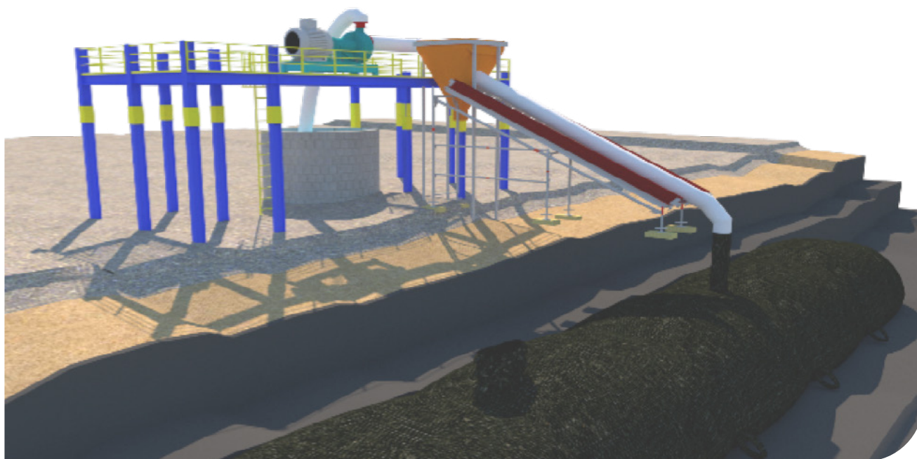
▲ Figura 17.5 | Llenado de Geotextile Tubes por gravedad.
