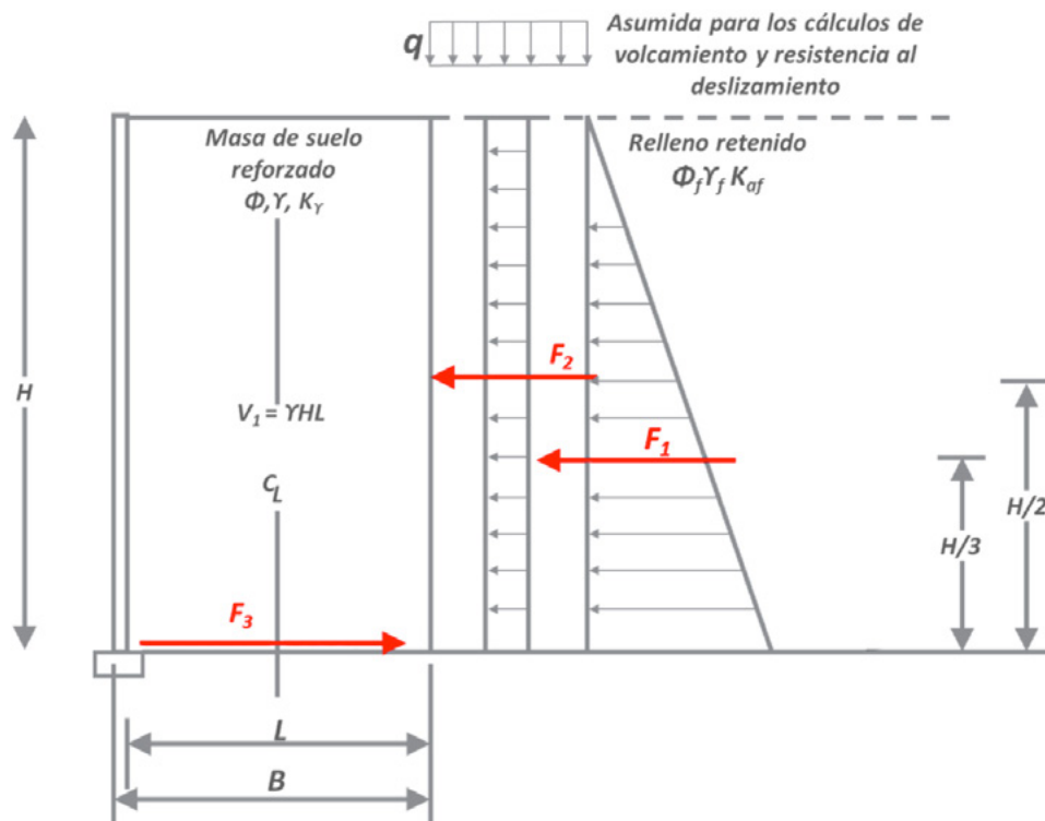
▲ Figura 11.10 | Análisis por Deslizamiento Estado Límite de Resistencia.
