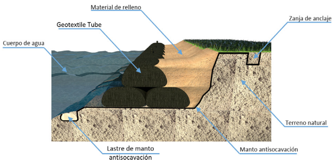
▲ Figura 17.4 | Solución compuesta por Geotextile Tubes.
