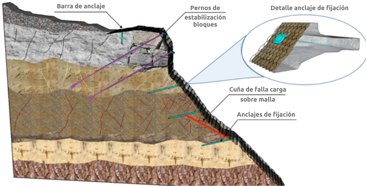
▲ Figura 16.9 | Elementos de fijación de la malla y elementos puntuales. Carga de material que soportará la malla.
