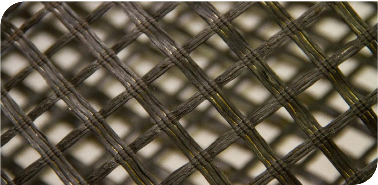
▲ Fotografía 2.11 | Geomalla Fibra de Vidrio.
