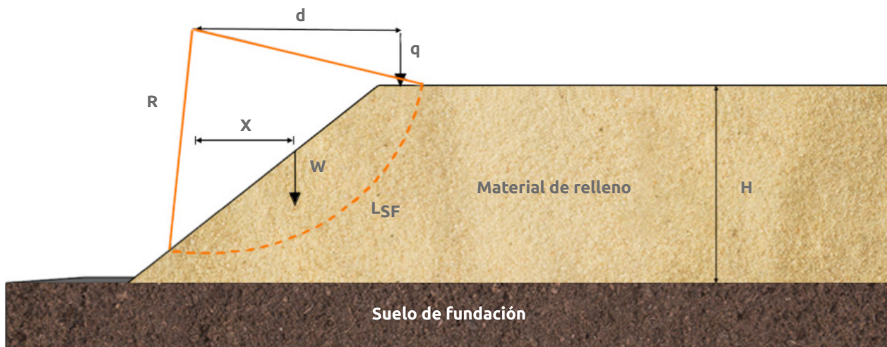
▲ Figura 12.4 | Esquema superficie de falla.
