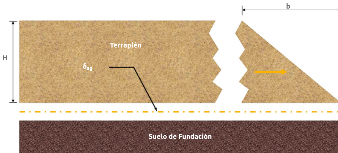
▲ Figura 13.8 | Desprendimiento lateral del talud.
