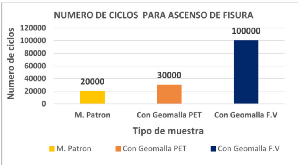
▲ Gráfico 8.4 | Comparación entre Geomallas para repavimentación en función de carga.
