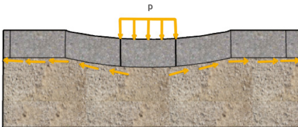
▲ Figura 4.8 (b) | Esquema del efecto membrana, deformación del suelo de fundación y activación de los esfuerzos por tensión en la interfase Geocelda – Geosintético de separación y material de fundación.
