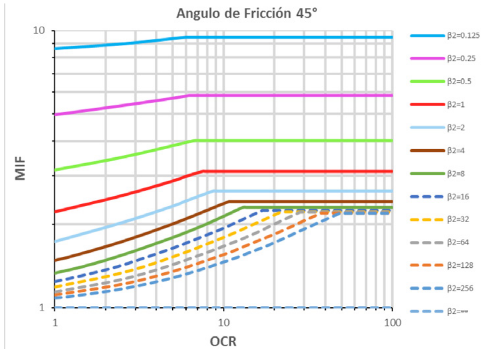
▲ Figura 7.8 d | Gráficos para la determinación de MIF en capas de suelo reforzadas con Geoceldas.
