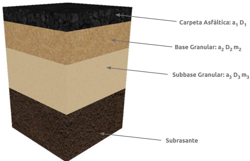
▲ Figura 6.4 | Sección de la estructura con sus respectivos coeficientes de capa.
