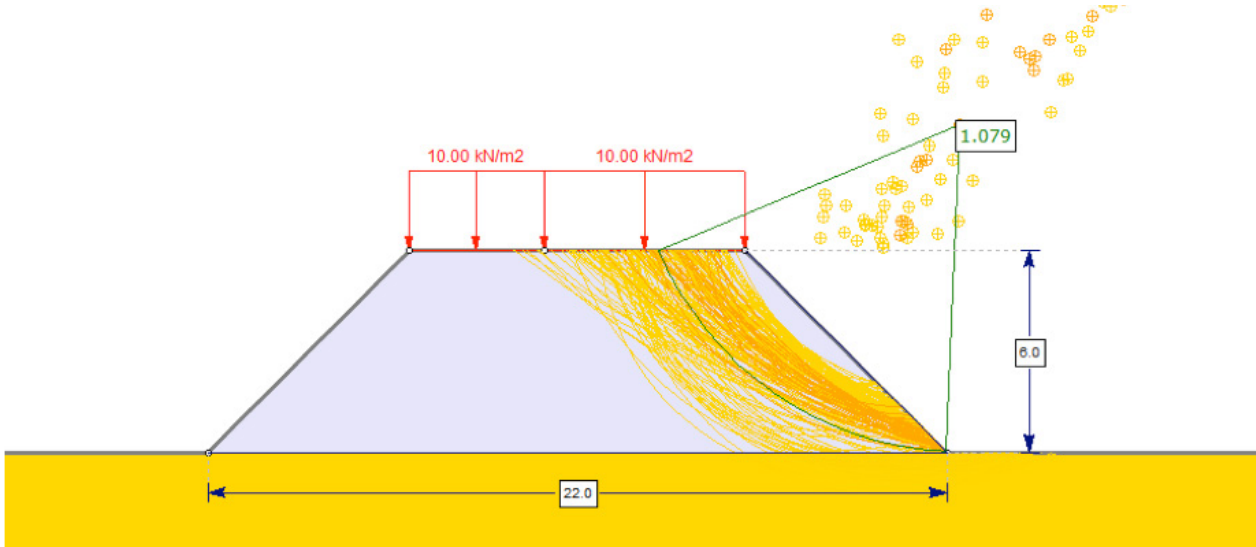
▲ Figura 12.2 | Resultado de un análisis de estabilidad a un talud sin refuerzo Realizado en Slide 7.0.
