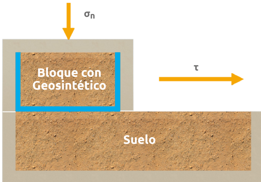
▲ Figura 2.8 | Ensayo fricción suelo-Geosintético.
