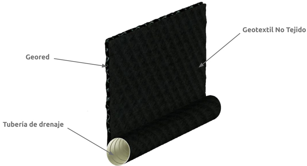
▲ Figura 2.6 | Geodrén Vial.
