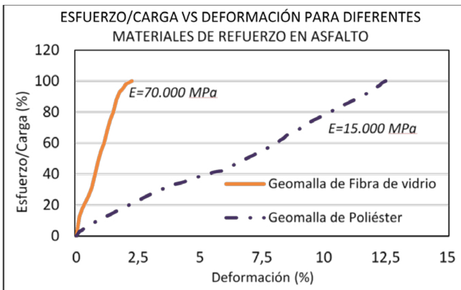
▲ Gráfico 8.5 | Comparación entre Geomallas para repavimentación en función del módulo.
