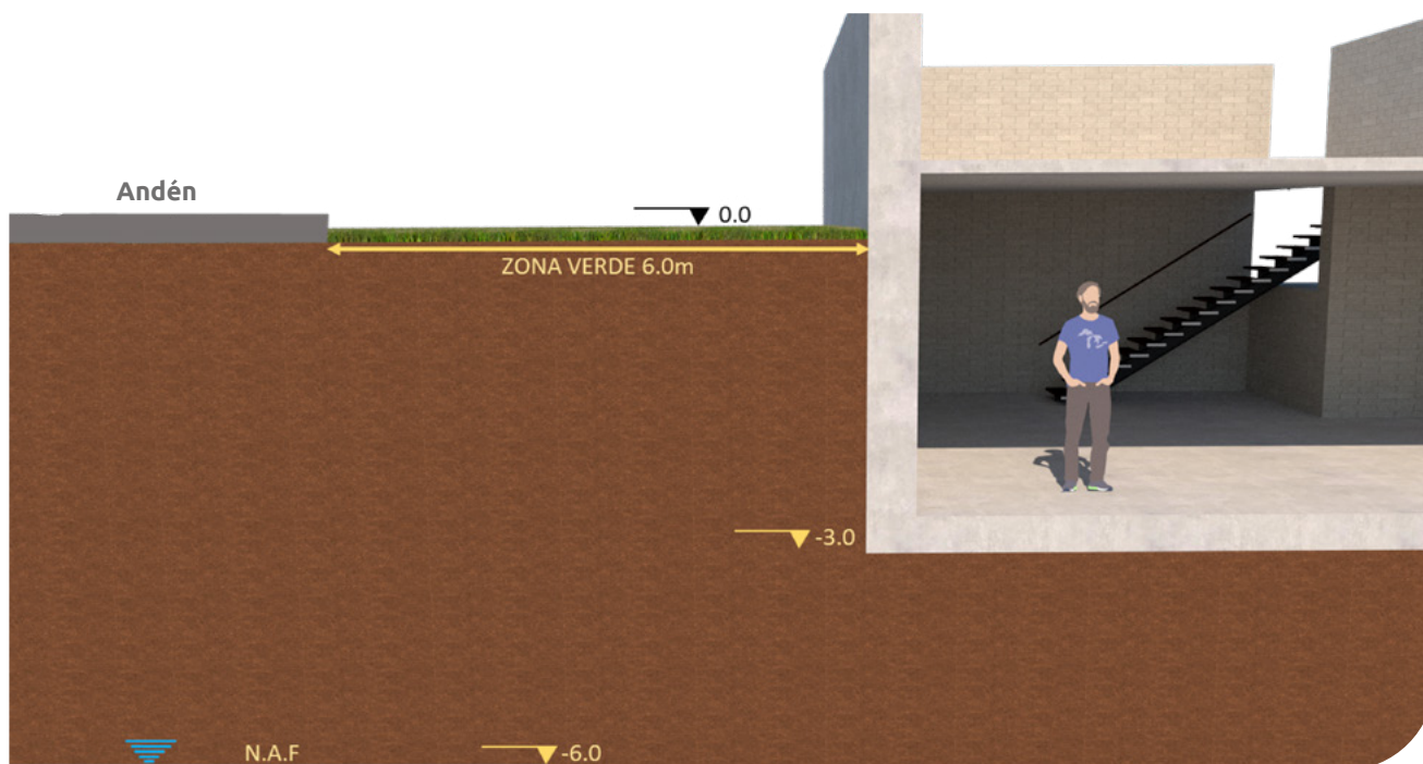
▲ Figura 10.24 | Esquema ejemplo sistema de sub-drenaje.
