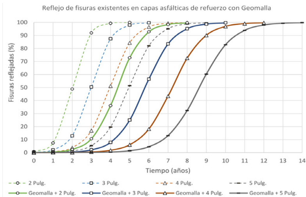
▲ Gráfico 8.8 | Porcentaje de fisuras reflejadas en el tiempo, en función del espesor del refuerzo, en pavimentos flexibles con el uso de Geomalla de Fibra de Vidrio como intercapa.
