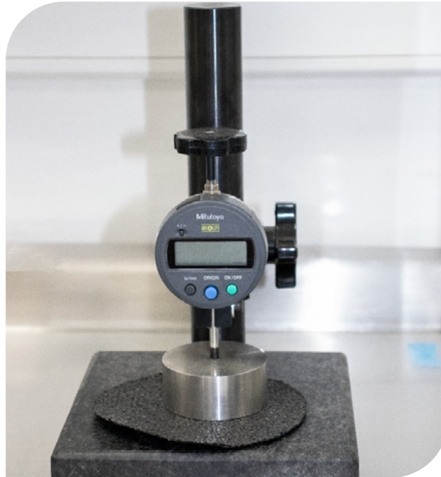
▲ Fotografía 2.28 | Ensayo espesor nominal.
