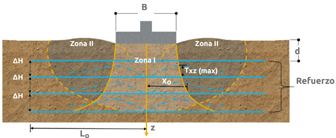
▲ Figura 14.6 | Mecanismo de falla en cimentaciones reforzadas.
