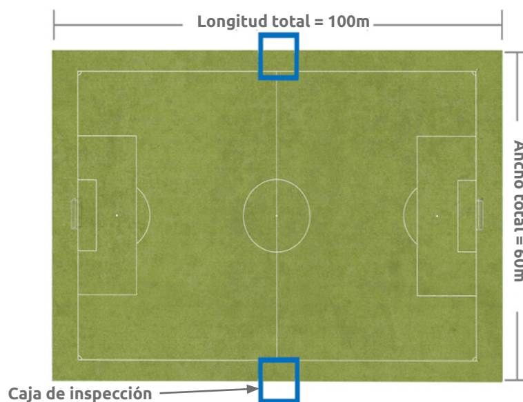
▲ Figura 10.20 | Dimensionamiento del ejemplo para campos deportivos.
