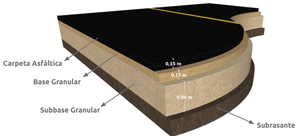
▲ Figura 5.7 | Estructura sin Geotextil de separación.
