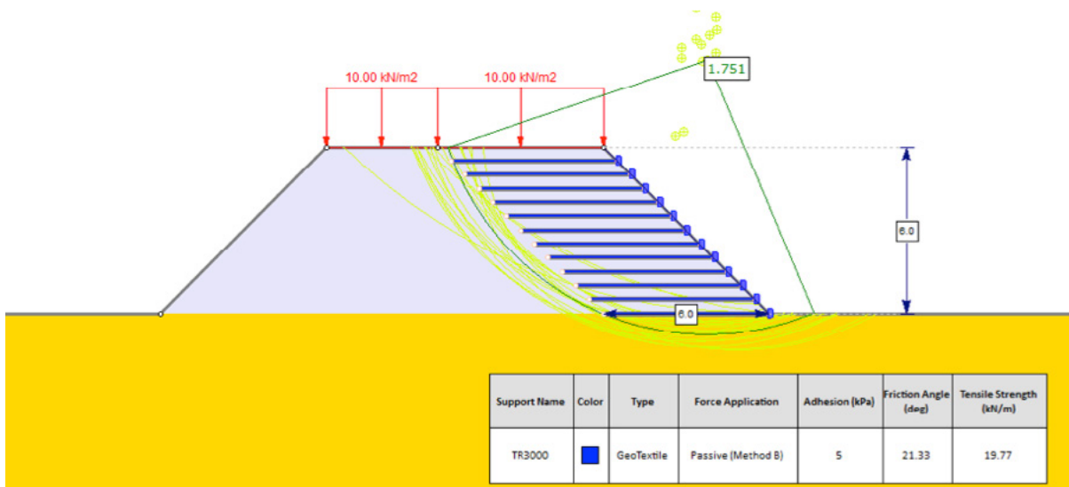
▲ Figura 12.3 | Resultado de un análisis de estabilidad a un talud con refuerzo Realizado en Slide 7.0.
