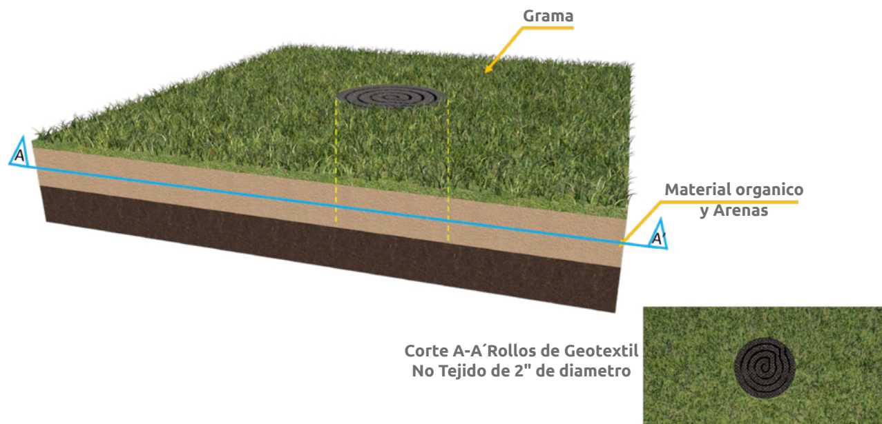
▲ Figura 10.10 | Sumideros para incremento de velocidad de respuesta del sistema de drenaje.
