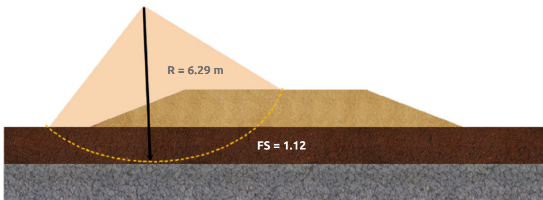
▲ Figura 13.14 | Cuña de falla a tener en cuenta para el diseño.
