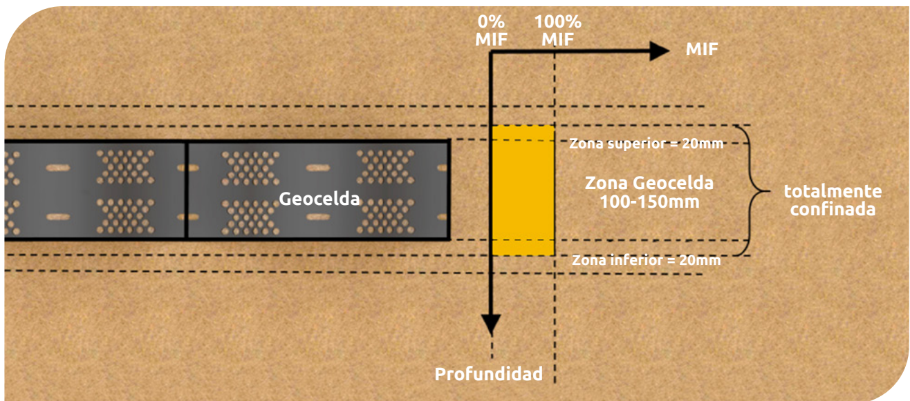
▲ Figura 7.13 | Distribución del confinamiento en la zona reforzada.
