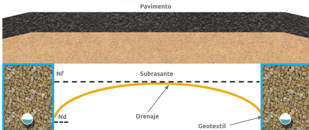
▲ Figura 9.8 | Sistema de subdrenaje lateral en carreteras.
