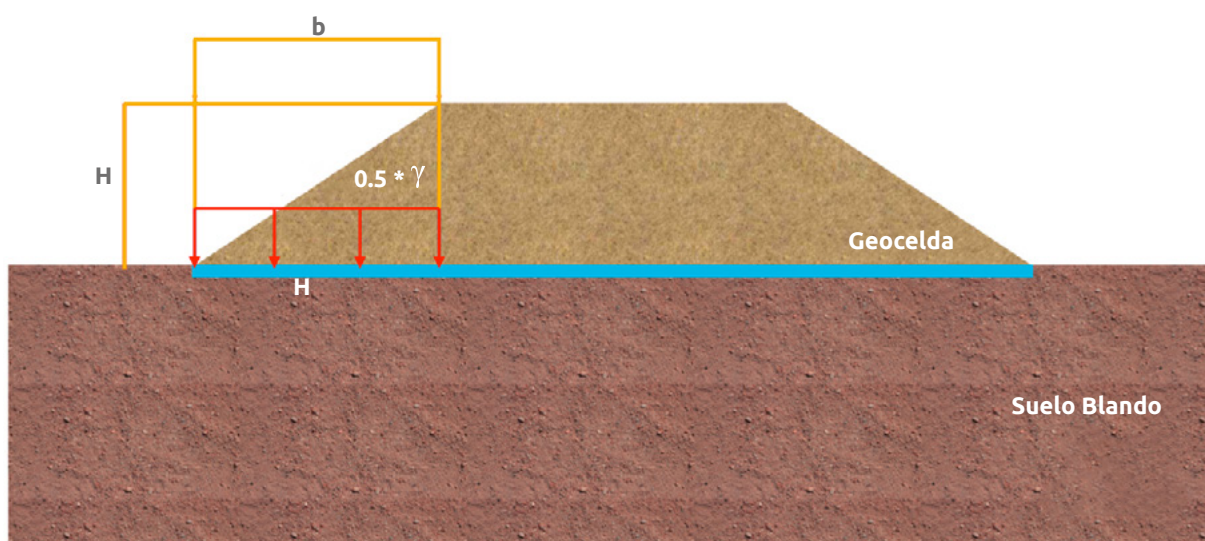
▲ Figura 13.11 | Refuerzo de terraplén con Geocelda.
