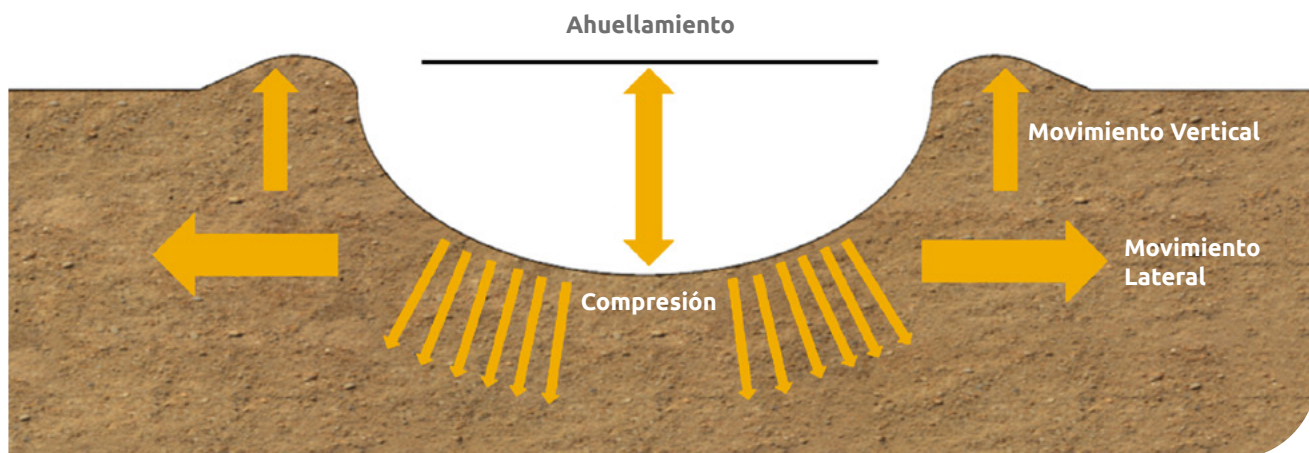
▲ Figura 4.12 | Ahuellamiento carretera no pavimentada.
