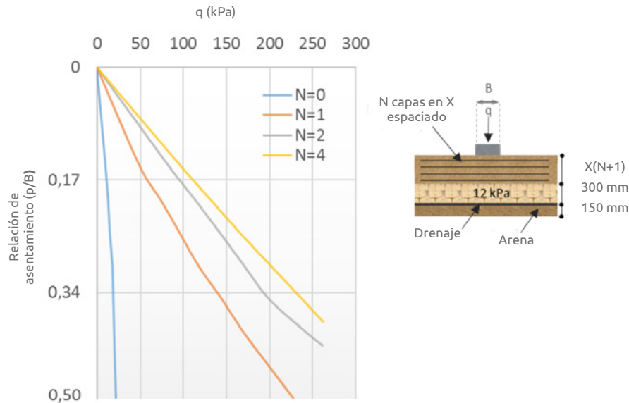
▲ Figura 14.1 | Prueba de carga cimentación reforzada con Geotextil.
