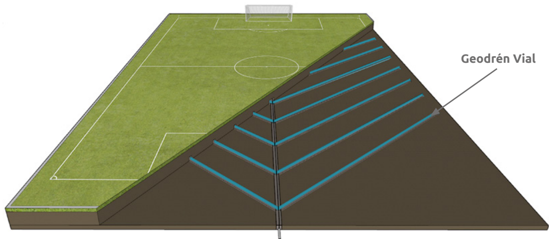
▲ Figura 10.5 | Subdrenaje en campos deportivos con Geodrén vial.
