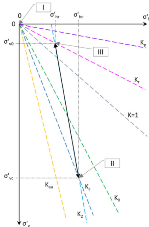
▲ Figura 7.7 | Gráfica de trayectoria de esfuerzos.
