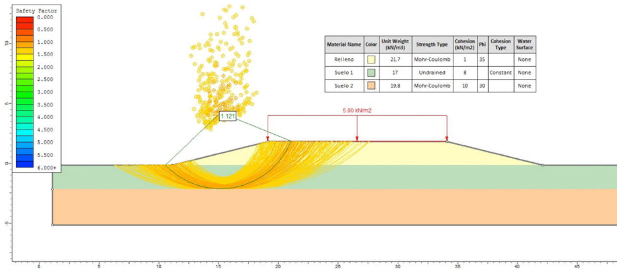
▲ Figura 13.13 | Análisis de estabilidad del terraplén sin refuerzo.
