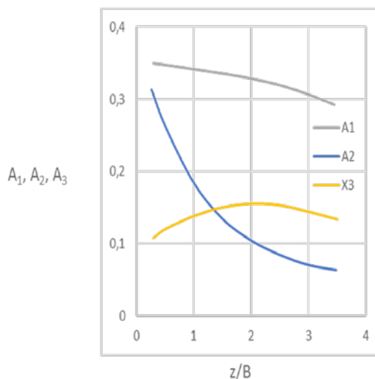
▲ Figura 14.10 | Variación de A_1 , A_2 , A_3 con respecto a z/B .
