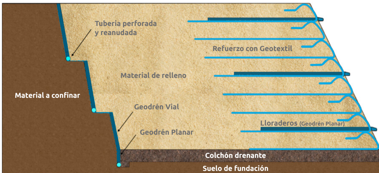
▲ Figura 12.6 | Esquema de obras de subdrenaje en un terraplén.
