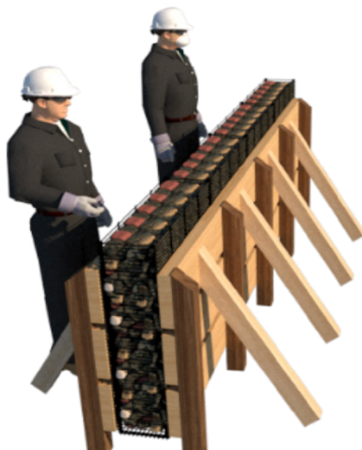
▲ Figura 17.16 | Uso de formaleta y llenado del Geocolchón.
