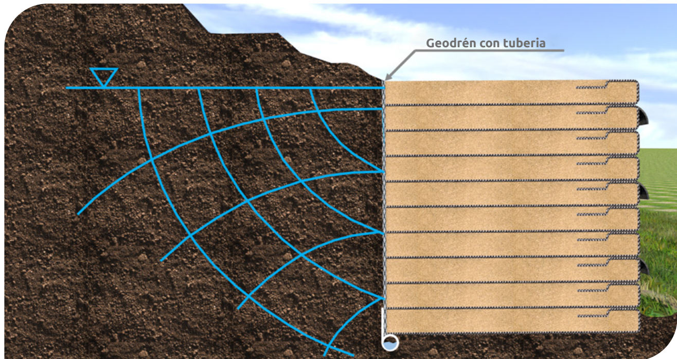
▲ Figura 10.23 | Muro de contención en suelo reforzado.
