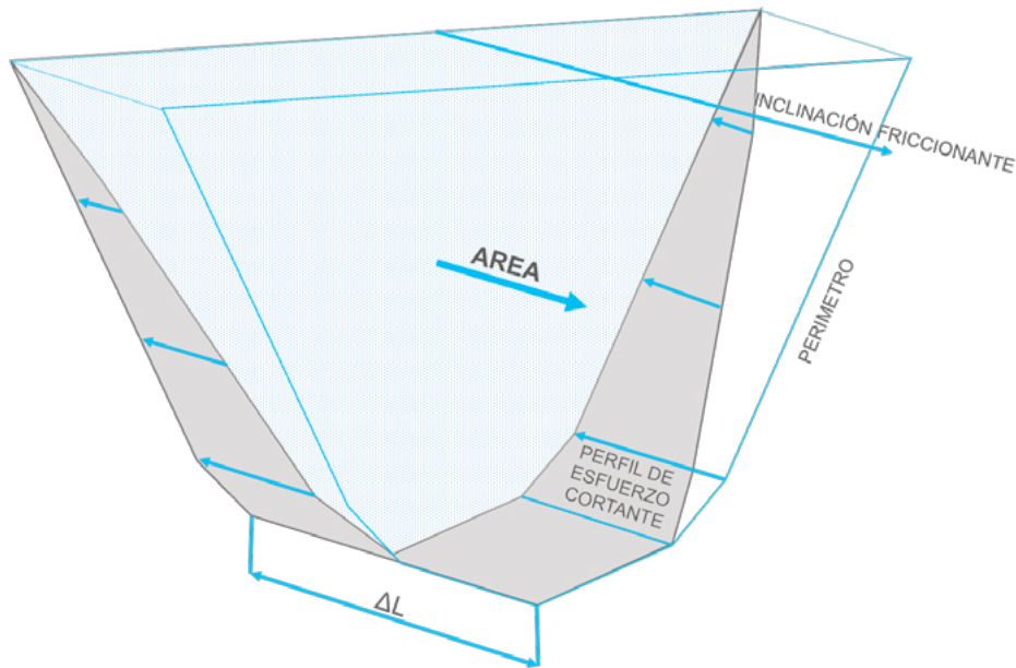
▲ Figura 16.4 | Esfuerzos sobre una sección de canal.
