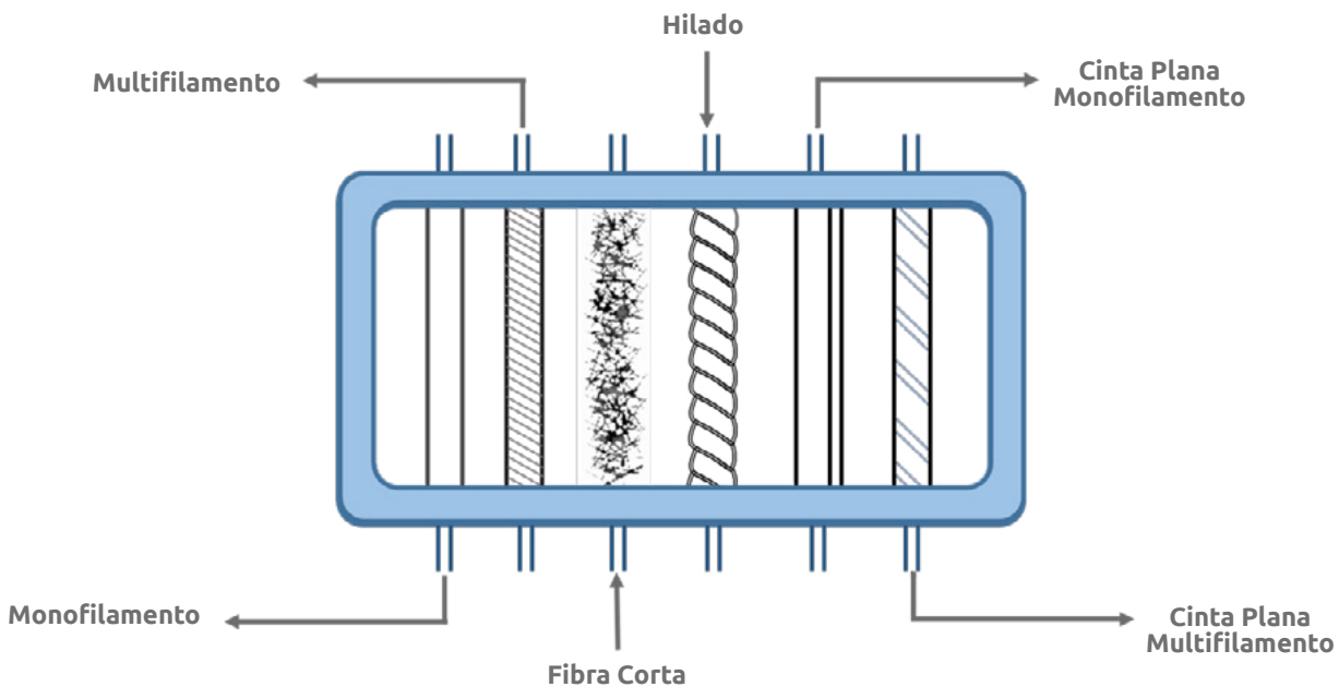
▲ Figura 2.1 | Tipos de fibras utilizadas en la construcción de Geotextiles.
