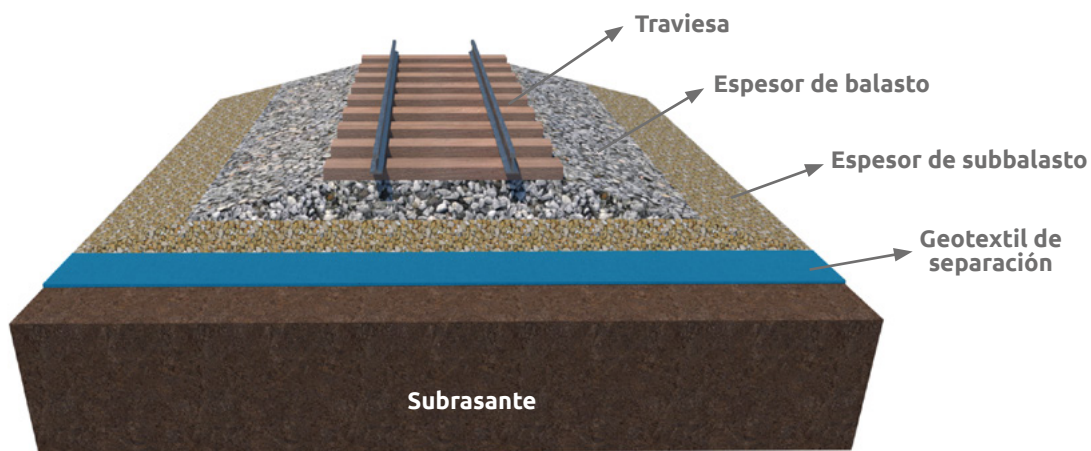
▲ Figura 5.9 | Separación en vías férreas.
