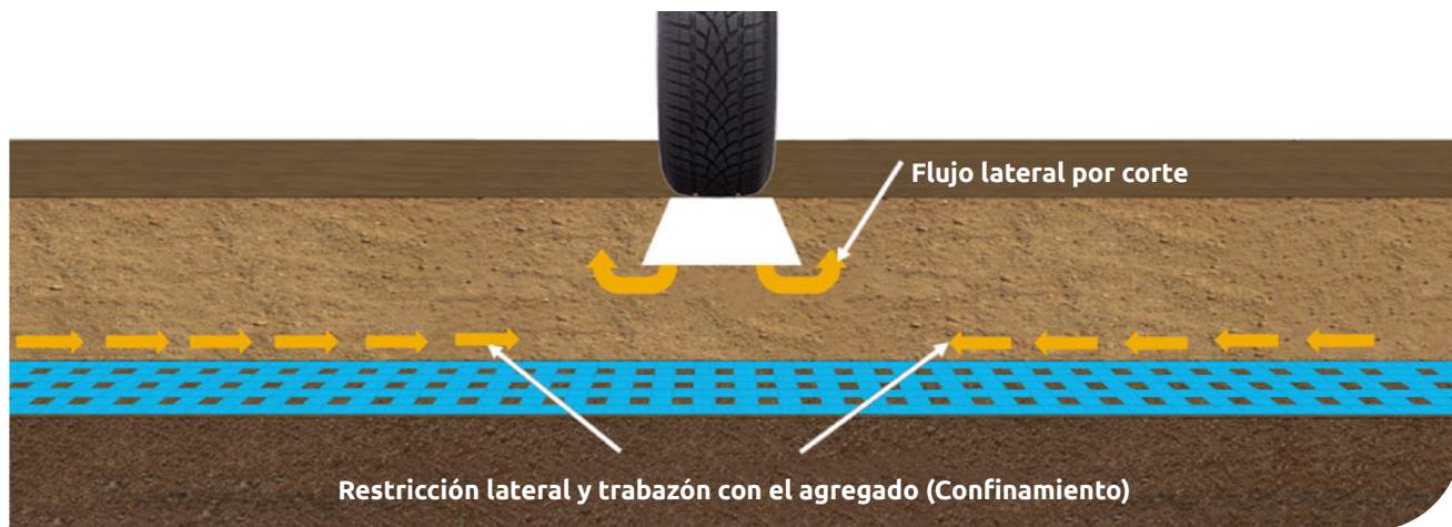
▲ Figura 4.3 | Confinamiento lateral generado por la Geomalla en un material granular.
