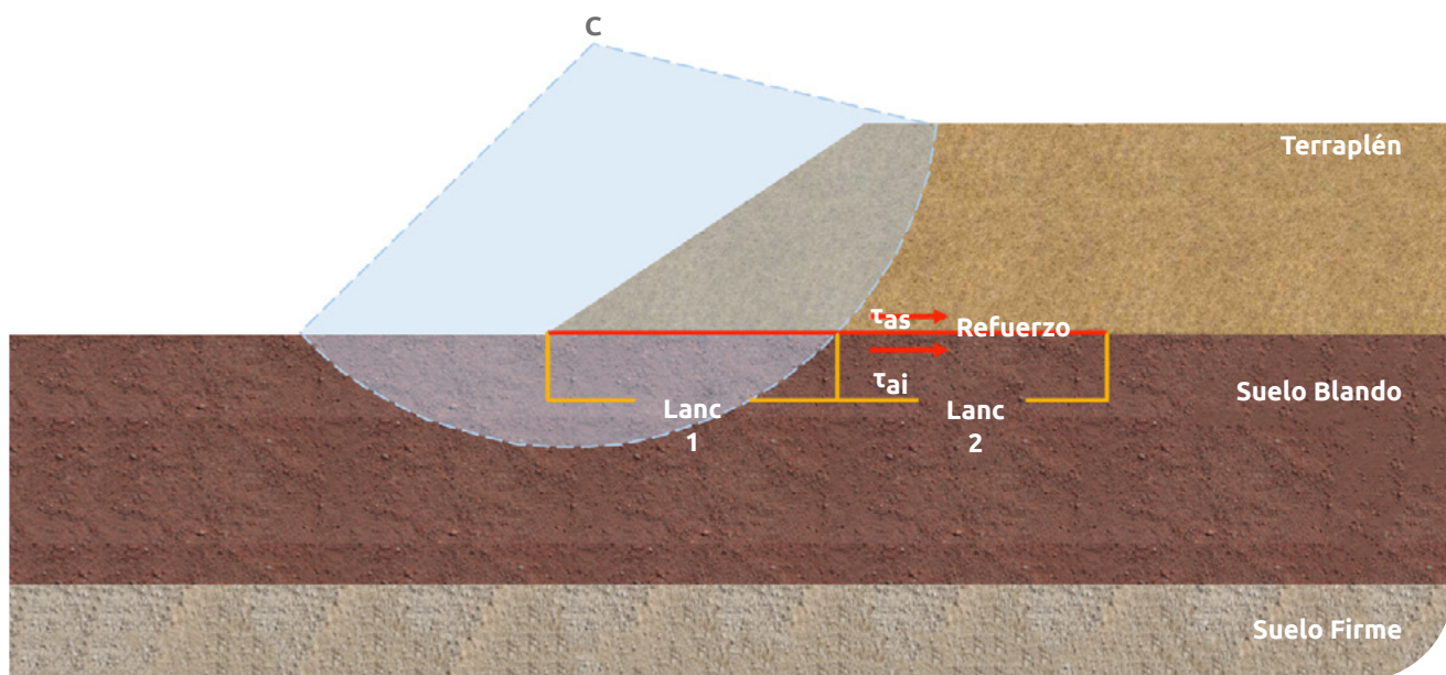
▲ Figura 13.2 | Longitud de empotramiento.
